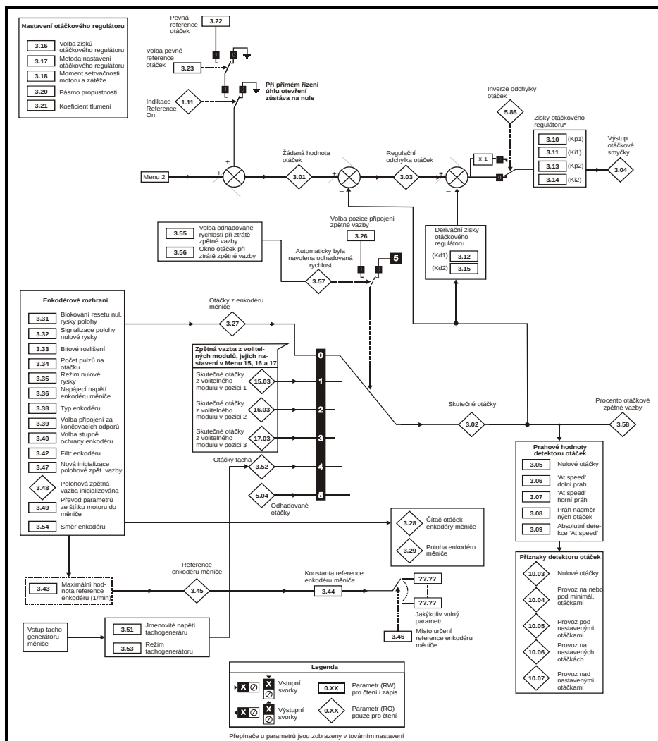
Obr. 8-3 Logický diagram Menu 3
