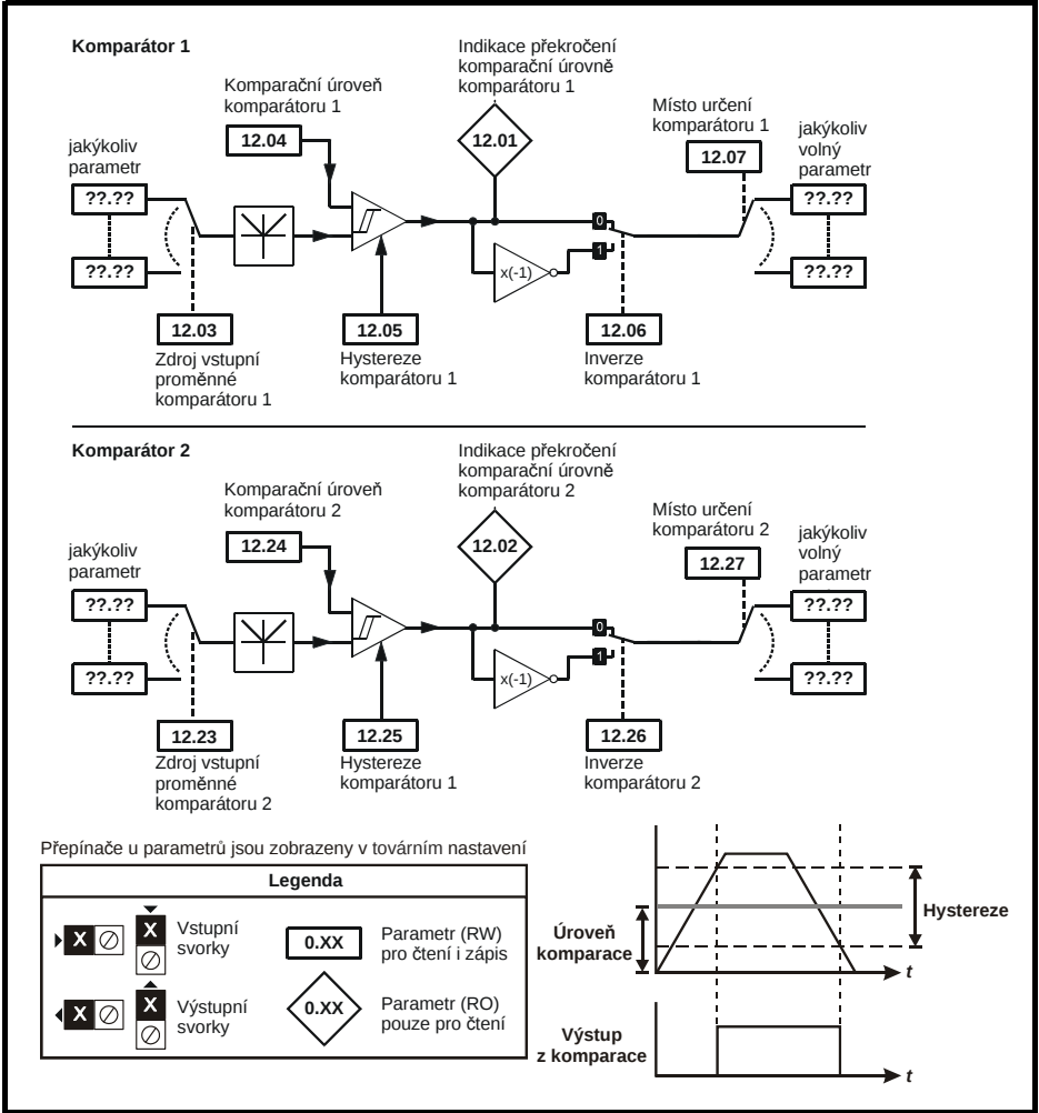
Obr. 8-14 Logický diagram Menu 12
