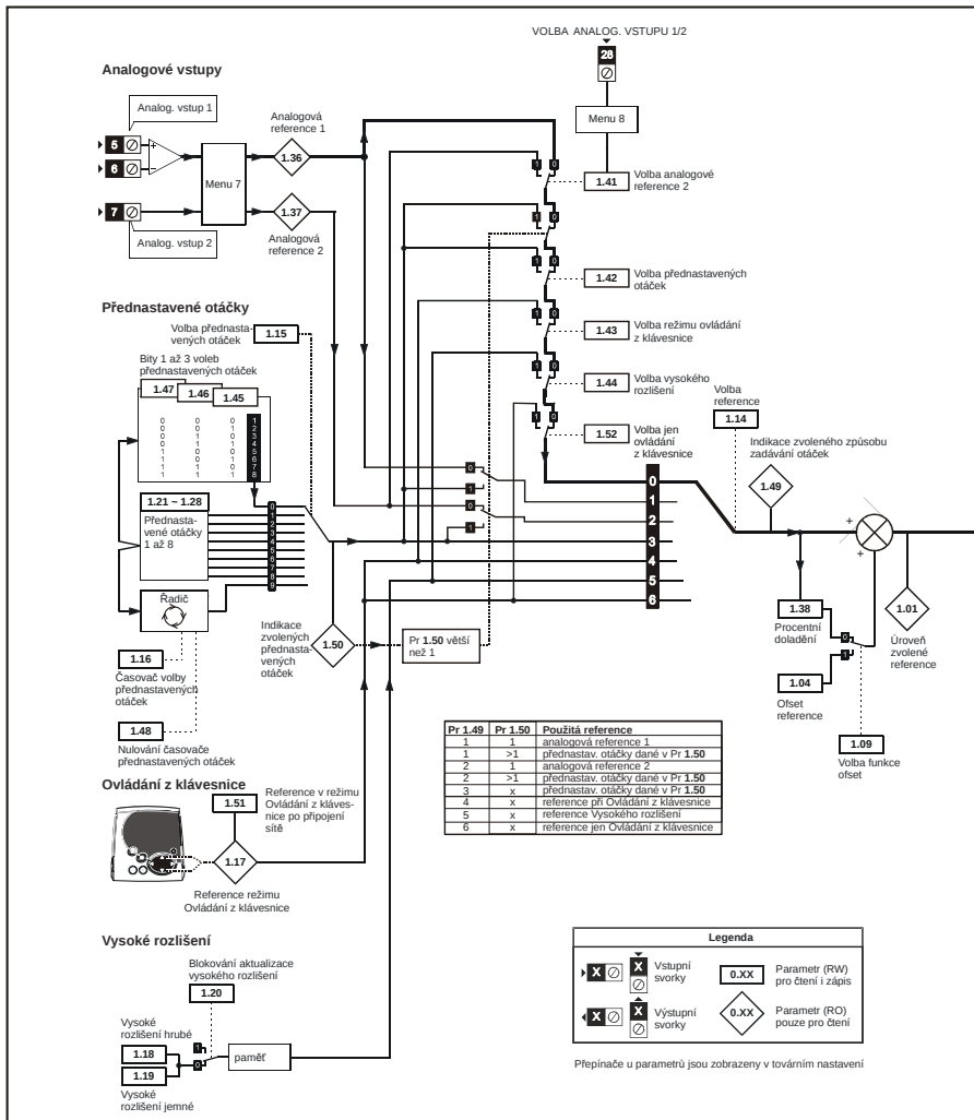
Obr. 8-1 Logický diagram Menu 1
